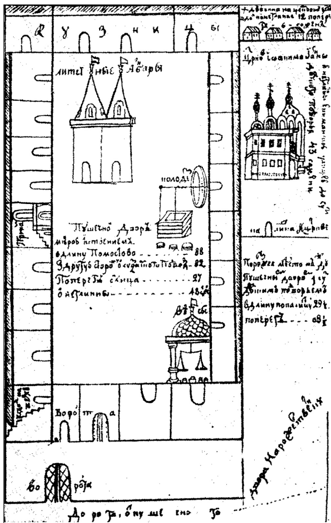
Пушечный двор в Москве во второй половине XVII в. Чертеж
